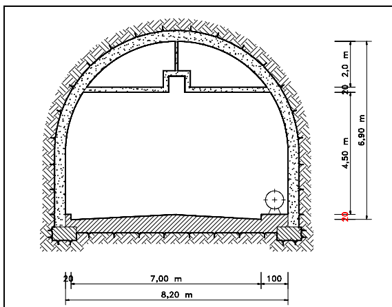
PŘÍČNÝ ŘEZ TUNELU PUŠKIN
