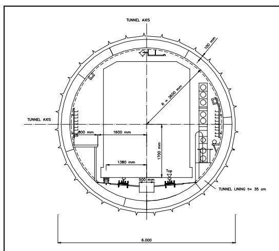
PŘÍČNÝ PROFIL 1 – TRÁŤOVÉ TUNELY (TBM)
