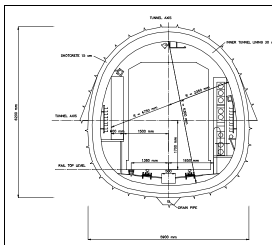
PROFIL 1 – TRÁŤOVÉ TUNELY (TBM)
