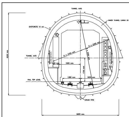
PRŮŘEZ 1 – TRAŤOVÉ TUNELY (TBM)
