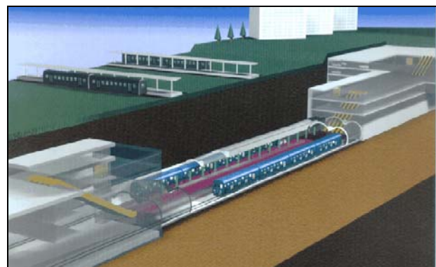
STANICE “FŐVÁM TER” – POČÍTAČOVÁ SIMULACE
